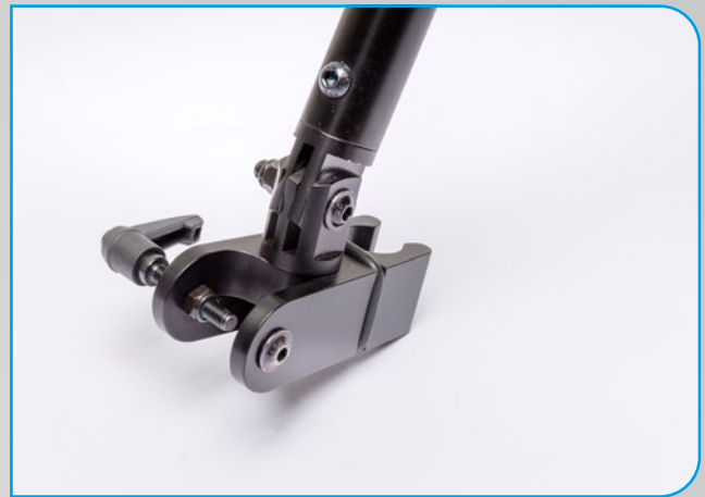
Befestigungsklemme für Rahmenrohrdurchmesser 23 mm mounting clamp for frame tube diameter 23 mm
